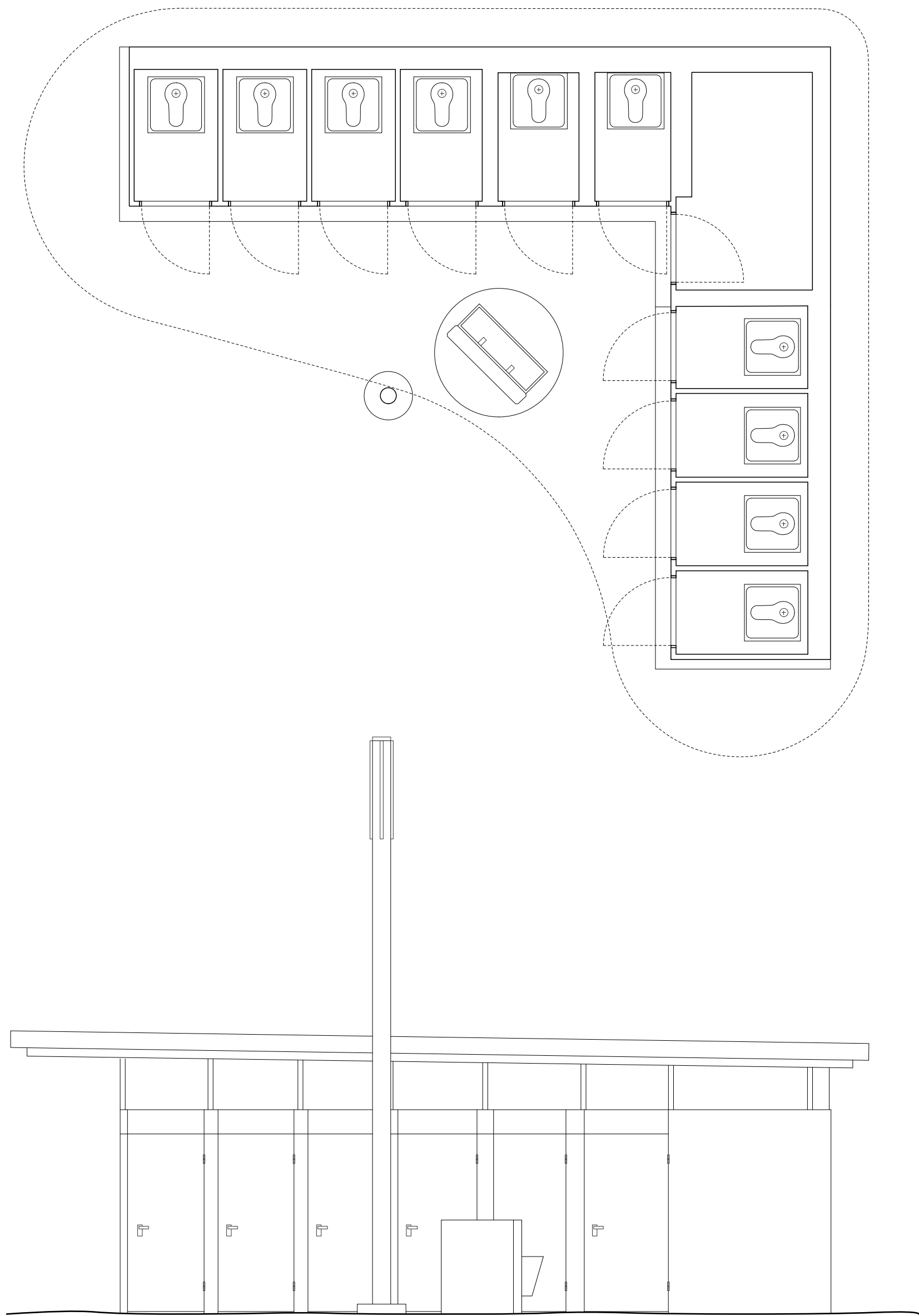
Toilettes, La Joux des Ponts (FR) 1:50
